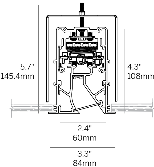
Recessed Bezel Trim (RBT)
