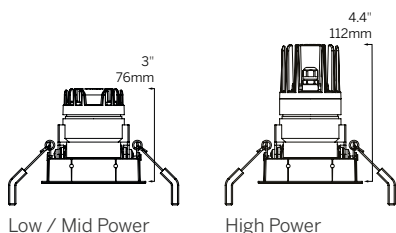
Recessed Bezel Trim (RBT)
