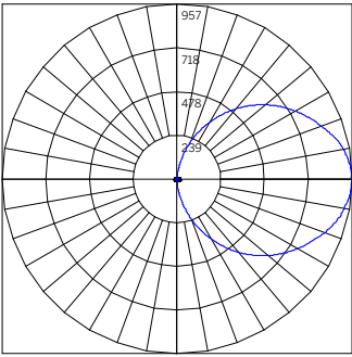
ISOILLUMINANCE - 48" OD M 3500K WG-CLWL-...-S-48-M-935-...-OD-W'
