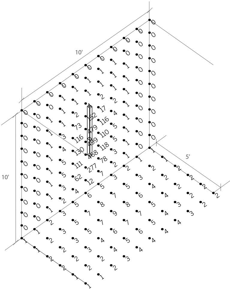
ISOILLUMINANCE - 48" OD M 3500K WG-CLWL-...-S-48-M-935-...-OD-W'
