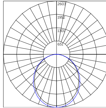
ILLUMINANCE - 48" OD P4 3000K WG-60LDL-...-S-48-930-P4-...-OD-W*
