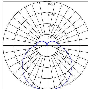
ILLUMINANCE - 48" DD P4 3000K WG-60LDL-...-S-48-935-P4-...-DD-W*
