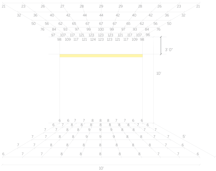
WG-20LWW-SRxT-...-S-...-H-935-OD-W 10'-0" ceiling height
