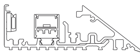
20 Linear Mini Edgeless Cove Plaster Trim
