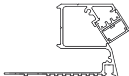
20 Linear Mini Z Cove Plaster Trim
