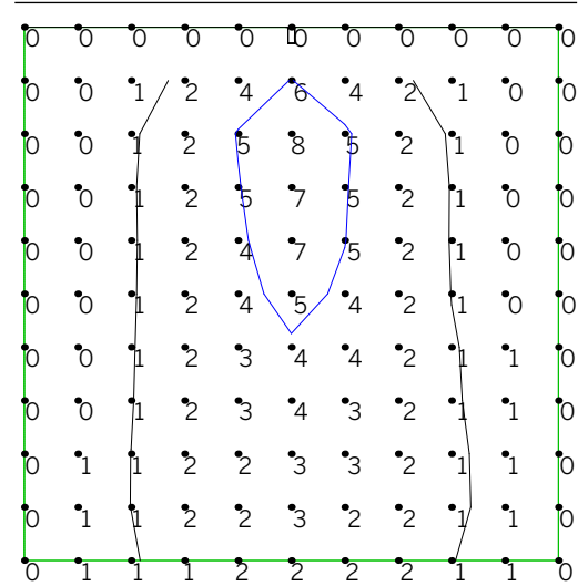
ISOILLUMINANCE DIAGRAM - MID POWER 3500K RWW WG-40SPTWW-...-M-92-35-...-SWW-WW-W 2
