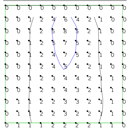
ISOILLUMINANCE DIAGRAM - MID POWER 3500K RWW WG-40RPTWW-...-M-92-35-...-RWW-WW-W 1,2
