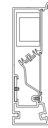
V Cove Bezel Trim
