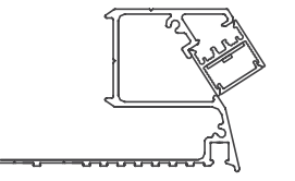
20 Linear Mini Z Cove Plaster Trim
