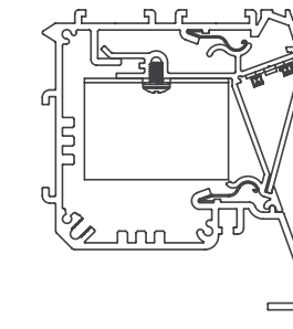
Z Cove Bezel Trim
