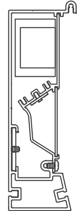
V Cove Bezel Trim
