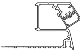
20 Mini Z Cove Plaster Trim
