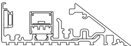
20 Mini Edgeless Cove Plaster Trim
