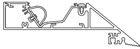
Mini Edgeless Cove Plaster Trim
