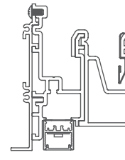
20LPF-SG-RBT Flush Bezel Trim Soft-graze
