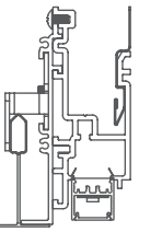
20LPF-RGT Flush Grid Trim
