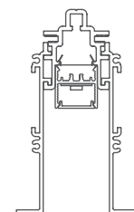
20LRR-RBT Recessed Bezel Trim
