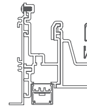
20LPF-SG-RBT Flush Bezel Trim Soft-graze 1·2·5
