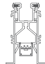
20LRF-RBT Flush Bezel Trim 1·2·3·4·5·6
