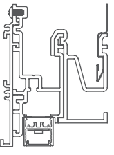
20LPF-SG-RRT Flush Return Trim Soft-graze 1·2·5
