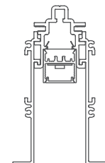
20LRR-RBT Recessed Bezel Trim 1·2·3·4·5
