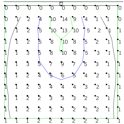
ISOILLUMINANCE DIAGRAM - HIGH POWER 3500K SWW WW 3 WG-75SPTWW-...-H-92-35-...-SWW-WW-W-W 4
