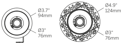
Bezel Trim (RBT)
