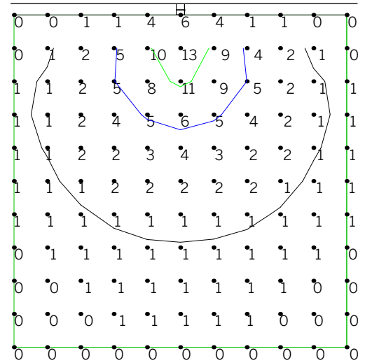
ISOILLUMINANCE DIAGRAM - HIGH POWER 3500K SAWW WW 3 WG-75SPTAWW-...-H-92-35-...-SAWW-WW-W-W 4
