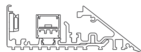
20 Mini Edgeless Cove Plaster Trim
