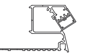
20 Mini Z Cove Plaster Trim
