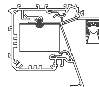
20 Z Cove Graze Bezel Trim
