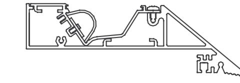
Mini Edgeless Cove Plaster Trim
