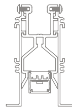
20 Linear Flush Bezel Trim
