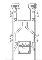
20 Linear Flush Bezel Trim
