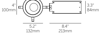
Recessed Bezel Trim (RBT)
