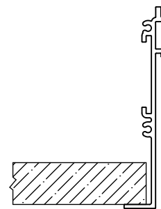
Bezel Trim
