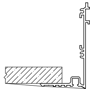
Trimless
