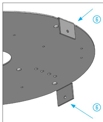
Baldachin Unterteil
