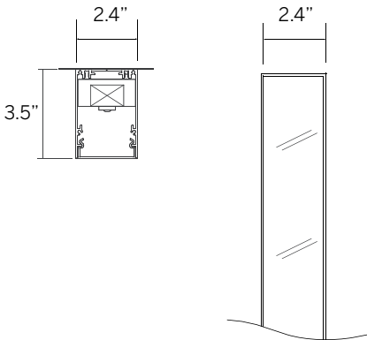
Flush Diffuser - OD / SD
